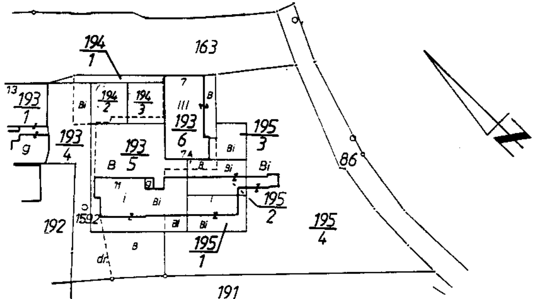
M A P A wyrys z mapy ewidencyjnej skala 1:1000
