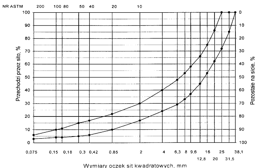
Rys. 1. Krzywe graniczne uziarnienia mieszanki mineralnej BA od 0 do 31,5 mm podbudowy drogi
