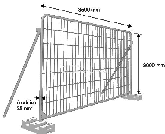
Rysunek poglądowy :płat odgradzający
